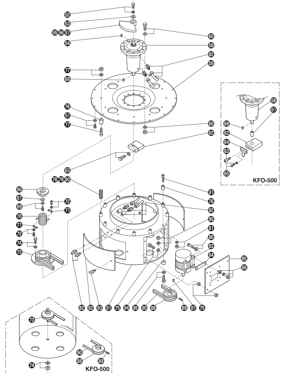
KFO 型分解構成図 (代表例: KFO-1000 型)
