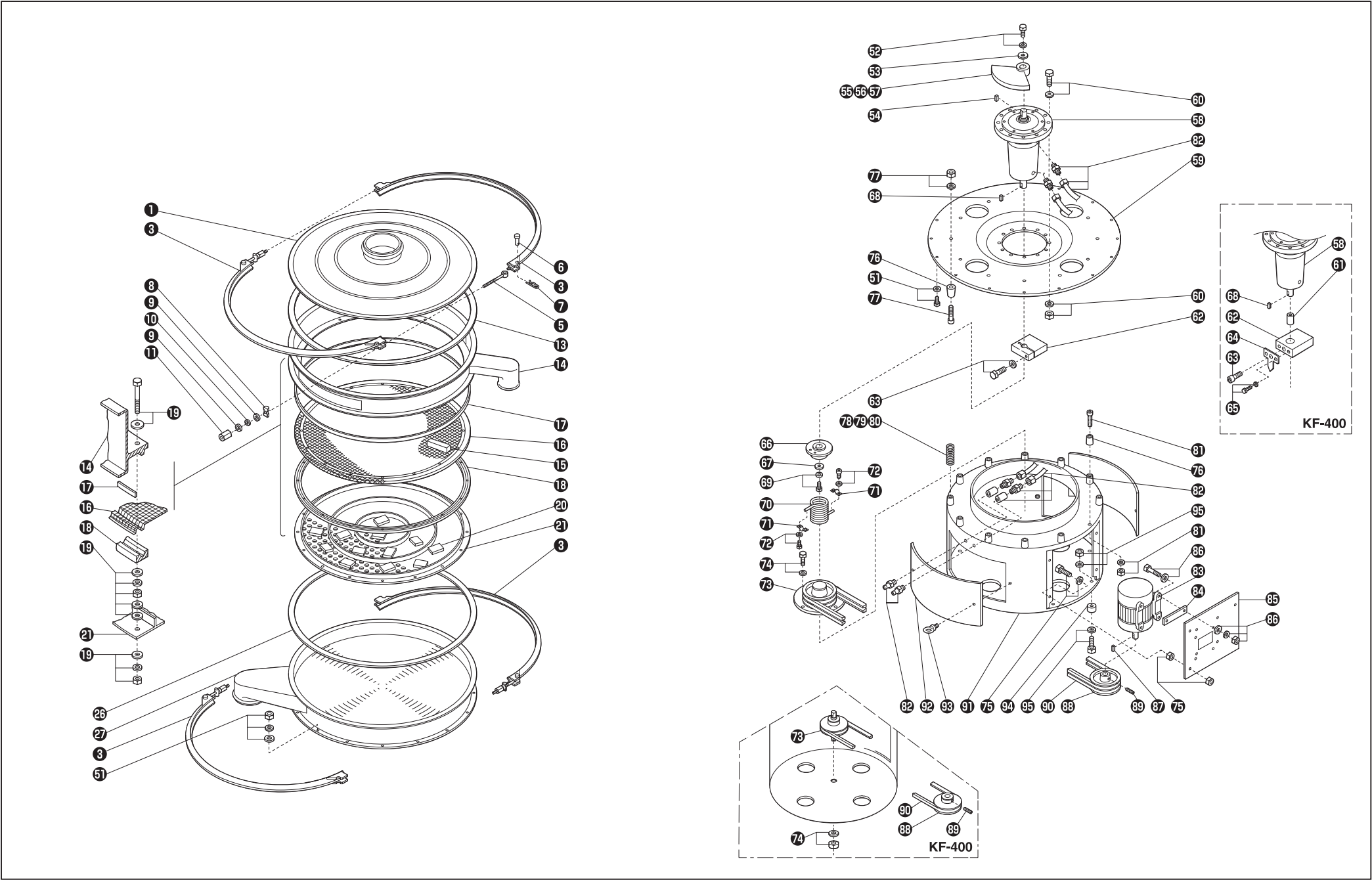
KF 型分解構成図 (代表例：KF-1000 型)
