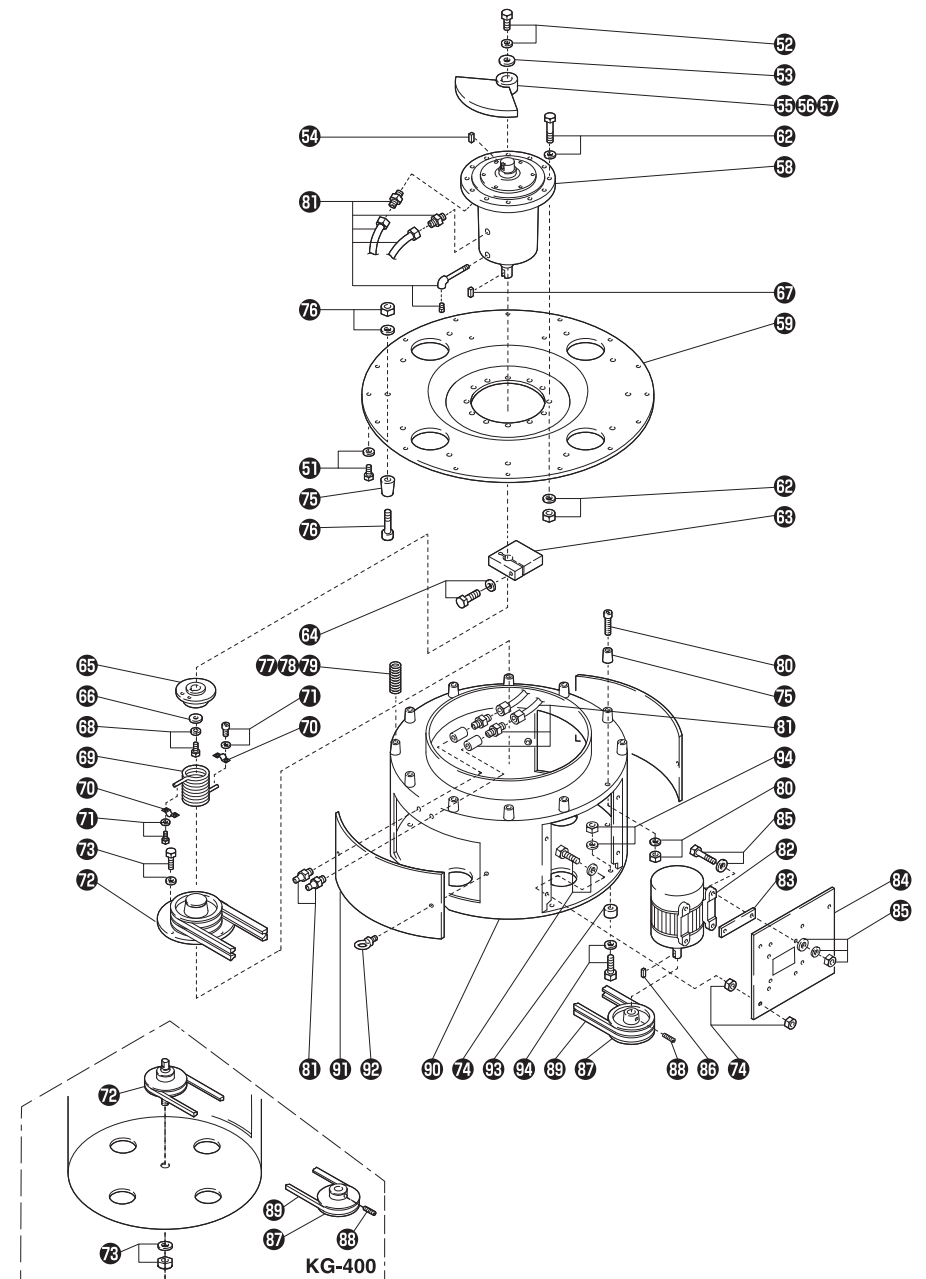
KG 型分解構成図（代表例：KG-1000 型）
