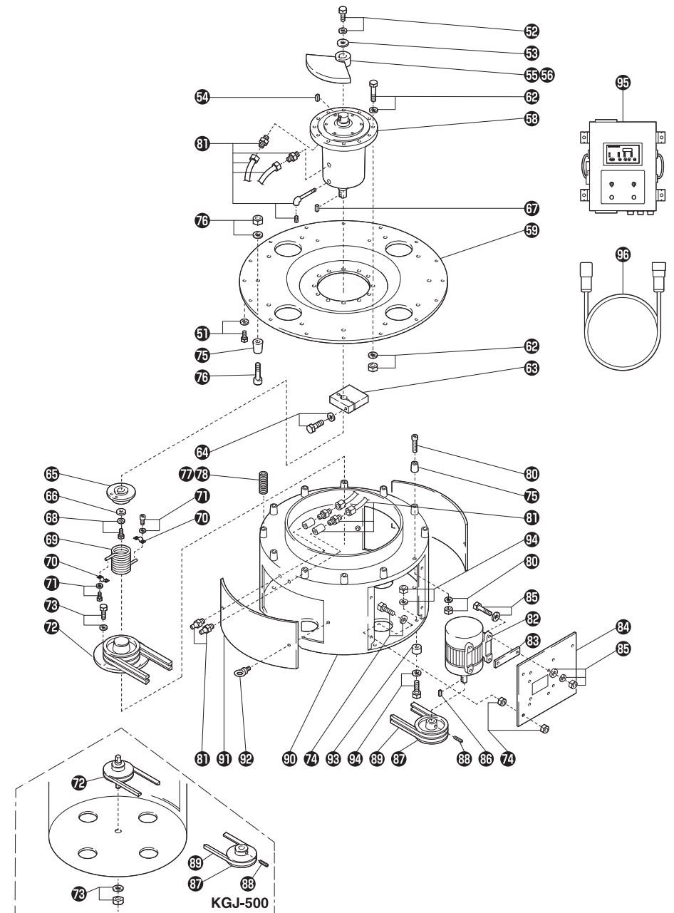
KGJ 型分解構成図（代表例：KGJ-1000 型）
