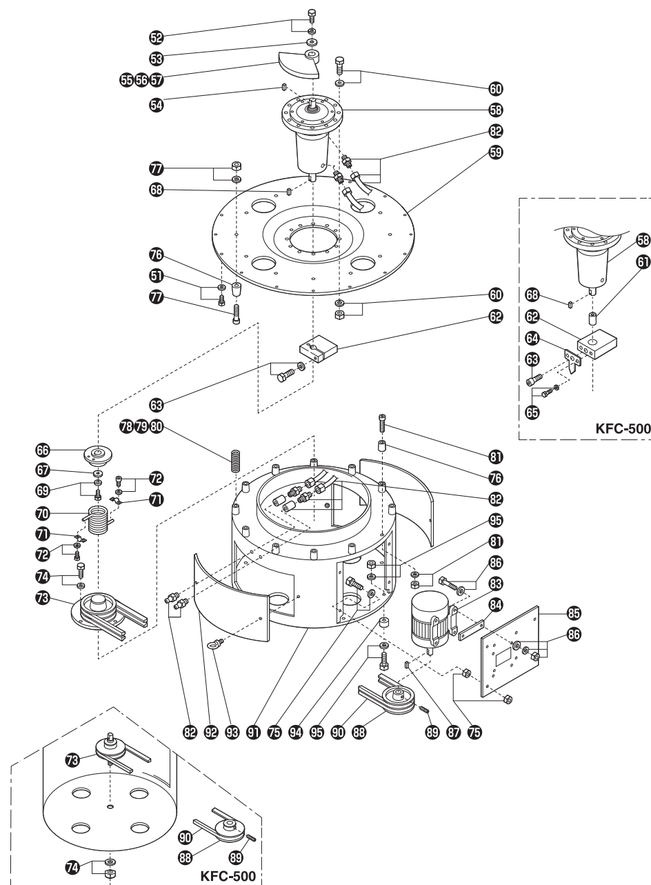
KFC 型分解構成図（代表例：KFC-1000 型）
